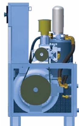
Автоматическая система натяжения ремня
