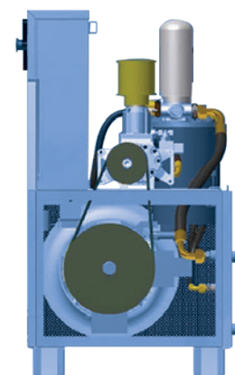
Sistema de tensado automático de la correa
