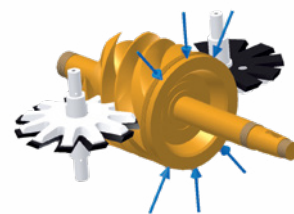
I carichi radiali agiscono sia sulla parte superiore che quella inferiore del rotore principale.
